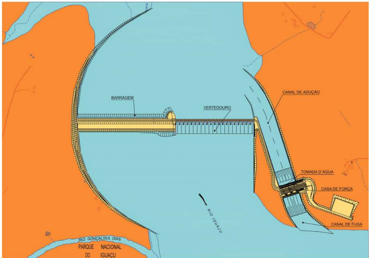
④ 2ª FASE DE CONSTRUÇÃO
