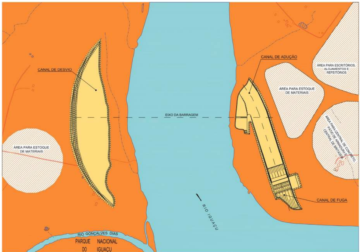
① 1ª FASE DE CONSTRUÇÃO
