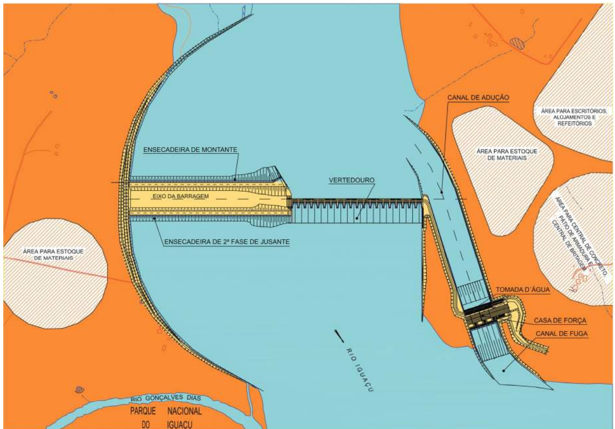
③ 2ª FASE DE CONSTRUÇÃO
