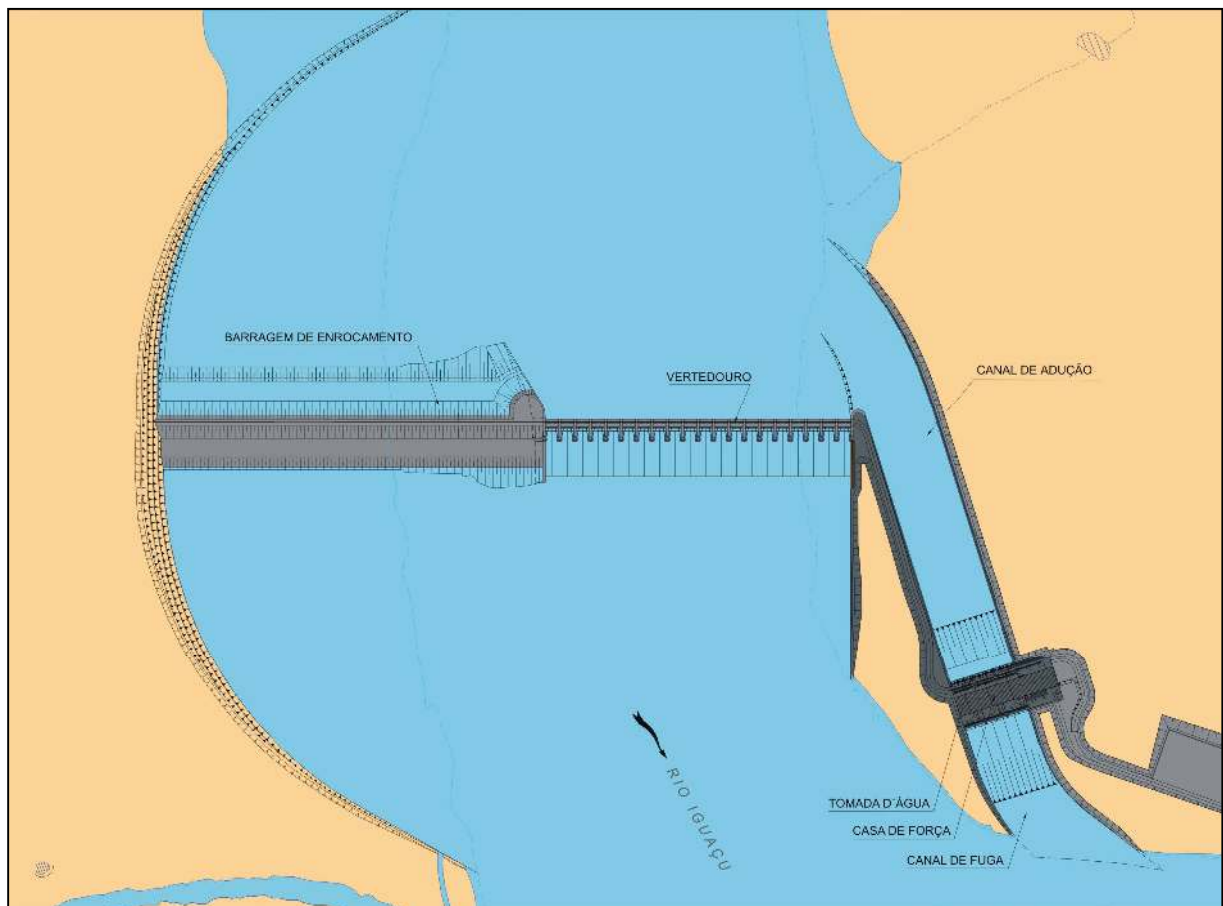
Figura 11 UHE Baixo Iguaçu - Alternativa de arranjo escolhida
