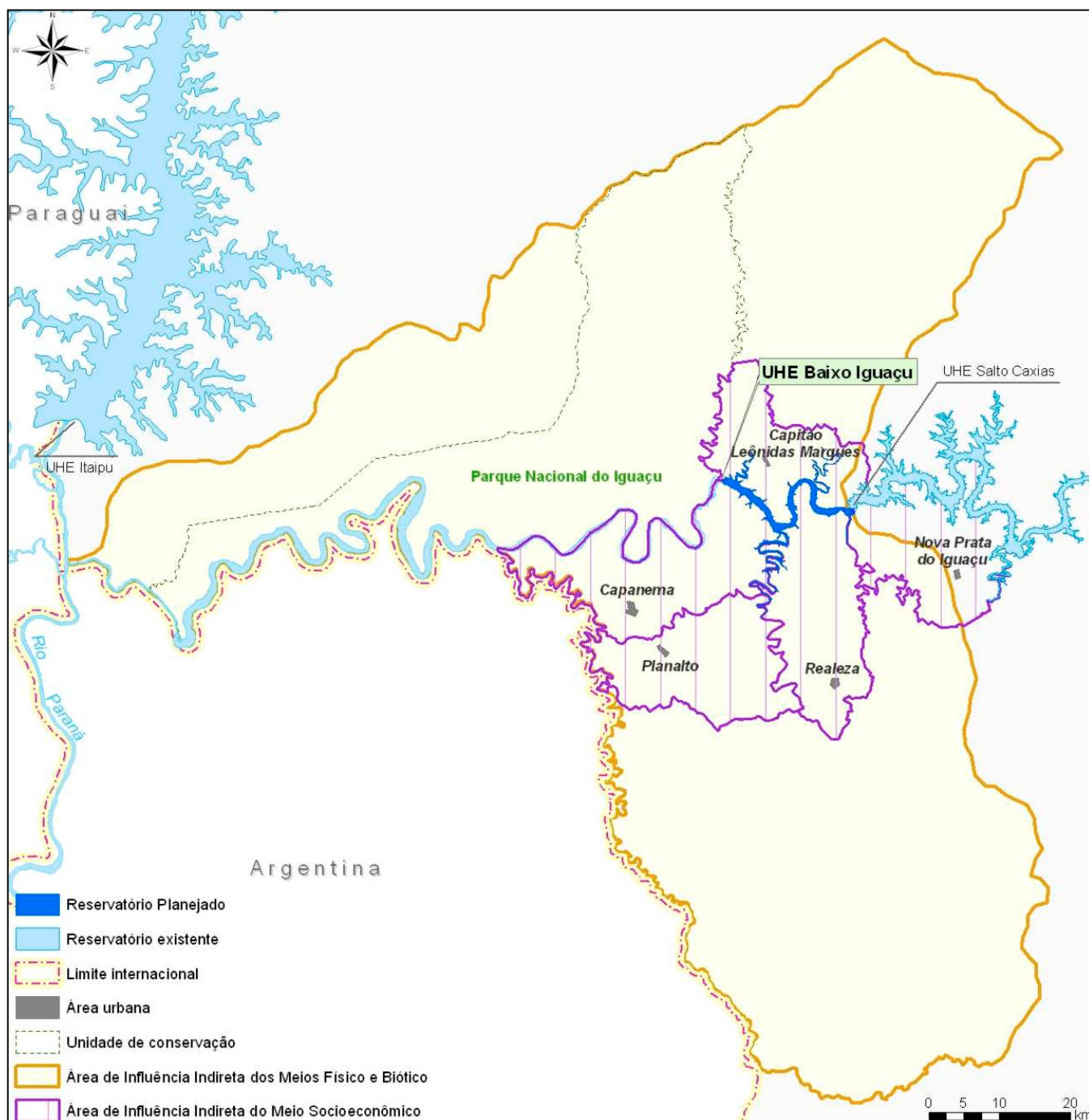
Figura 12 UHE Baixo Iguaçu - Áreas de influência
