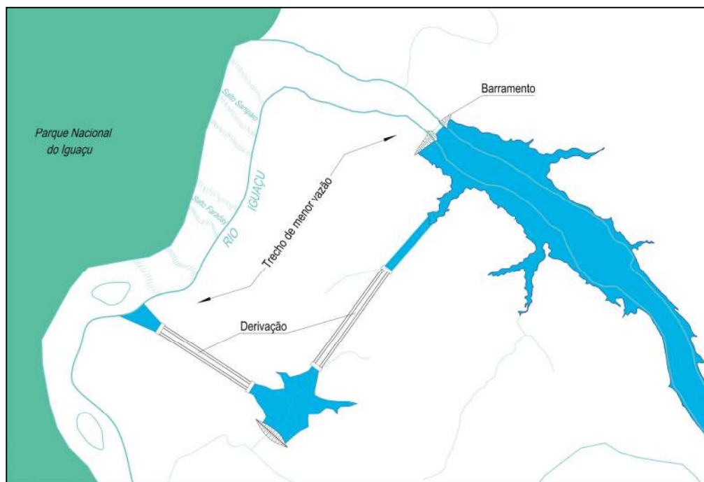
Figura 8 UHE Baixo Iguaçu - Alternativa de derivação longa
