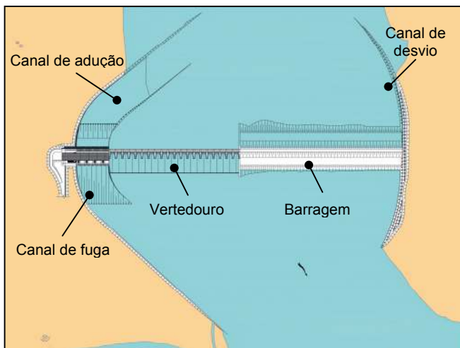
(a) Estruturas na margem direita e barragem na margem esquerda
