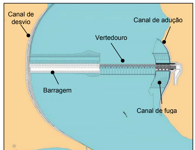
(b) Estruturas na margem esquerda e barragem na margem direita
