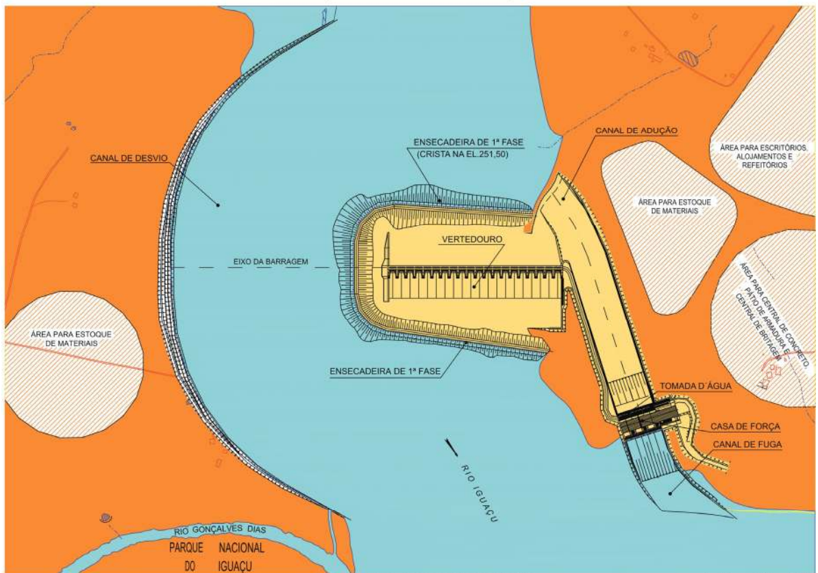
② 1ª FASE DE CONSTRUÇÃO
